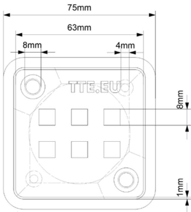
Draufsicht
