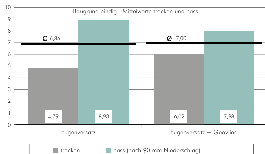
Abb. 5: Bleibende Setzung in mm nach Plattendruck mit 0,05 kN/cm 2 Bodenpressung (Vergleich: PKW-Auflast ~ 0,02 kN/cm 2 )
